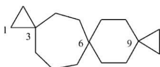
trispiro[2.2.2.2 9.2 6.3 3 ]heksadekan (PIN) poprawna
