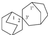
spiro[bicyklo[2.2.2]oktano-2,3'-bicyklo[3.2.1]oktan] (PIN) [bicyklo[2.2.2]oktan jest wymieniany przed bicyklo[3.2.1]oktan]
