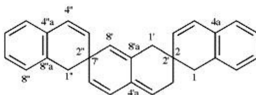
1H,1'H,1''H,3'H-2,2':7',2''-dispiroter[naftalen] (PIN)
