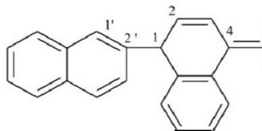
[1,2'-binaftaleno]-4(1 H )-yliden (preferowany przedrostek) [1,2'-binaftylo]-4(1 H )-yliden
