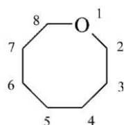
oksokan (PIN)
