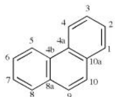
fenantren (PIN) (secialne numerowanie)
