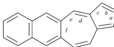
nafto[2,3- f ]azulen (PIN) [azulen (pierścienie 7, 5) preferowany względem naftalenu (pierścienie 6, 6)]
