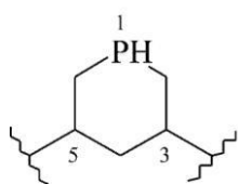
fosfino-3,5-diyl (preferowany przedrostek)
