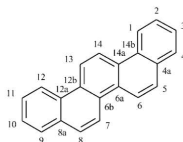
(6) picen (PIN)
