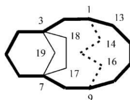
tetracyklo[7.4.3.2 3,7 .1 3,7 ]nonadekan (PIN)
