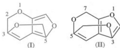
2 H -3,5-(epoksymetano)furo[3,4- b ]piran (PIN) (I) (nie 7 H -3,5-(epoksymetano)furo[2,3- c ]piran) (II) [preferowany układ pierścieni patrz P-25.4.3.4.2(d)]
