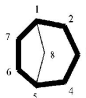
główny pierścień siedmioczłonowy
