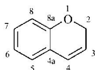
(23) chromen (pokazano izomer 2 H ) 1-benzopirany (pokazano izomer 2 H ; PINem jest: 2 H -1-benzopirany)
