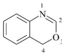
4 H -3,1-benzoksazyna (PIN) 4 H -benzo[ d ][1,3]oksazyna 4 H -3,1-benzooksazyna
