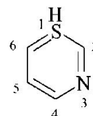
1 \lambda^4 ,3-tiazyna (PIN)
