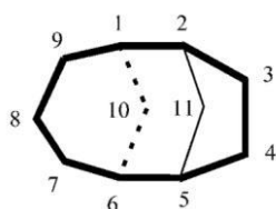
tricyklo[4.3.1.1 2,5 ]undekan (PIN) poprawnie
