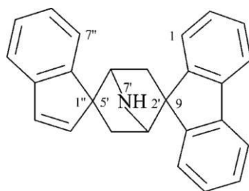
7'-azadispiro[fluoreno-9,2'-bicyklo[2.2.1]heptano-5',1''-inden] (PIN)
