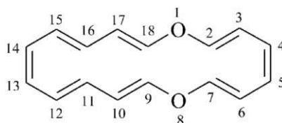
1,8-dioksacyklooktadecyn
