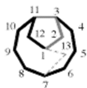
tricyklo[5.5.1.0 3,11 ]tridekan poprawnie
