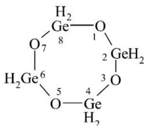
cyklotetragermoksan 1,3,5,7,2,4,6,8-tetroxatetragermokan (nazwa wstępnie wybrana, patrz P-12.2)
