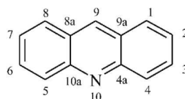
(4) akrydyna* (PIN) (specjalne numerowanie)
