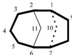
tricyklo[5.2.1.1 2,6 ]undekan niepoprawnie
