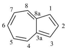
azulen (PIN)
