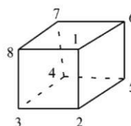
kuban (PIN) pentacyklo[4.2.0.0 2,5 .0 3,8 .0 4,7 ]oktan
