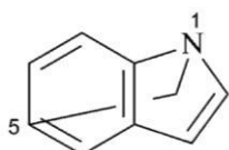
1,5-metanoindol (PIN)
