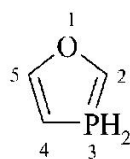
1,3 \lambda^5 -oksafosfol (PIN)
