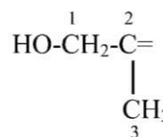
1-hydroksypropan-2-yliden (preferowany przedrostek) 2-hydroksy-1-metyloetyliden
