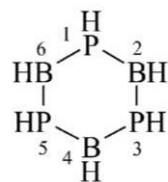
cyklotriborafosfan 1,3,5,2,4,6-trifosfatriborinan (nazwa wstępnie wybrana, patrz P-12.2)
