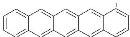
pentacen (PIN)
