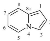
(20) indolizyna* (PIN)
