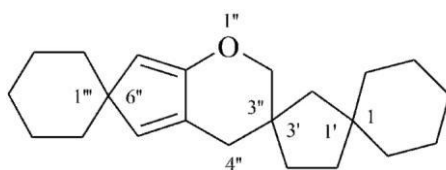
2''H,4''H-trispiro[cykloheksano-1,1'-cykloheksano-3',3''-cyklopenta[b]piran-6'',1'''-cykloheksan] (PIN)
