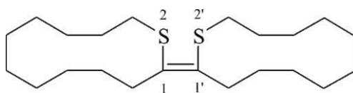
2,2'-ditia-1,1'-bi(cykłododecyliden) (PIN)
