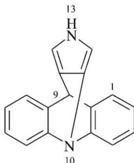
9H,13H-9,10-[3,4]epiapiroloakrydyna (PIN)
