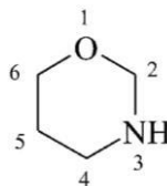
1,3-oksazynan (PIN)
