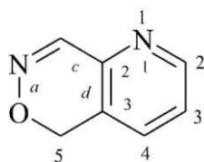
5 H -pyrido[2,3- d ][1,2]oksazyna (PIN) [oksazyna (2 heteroatomy) preferowana względem pirydyny (1 heteroatom)]
