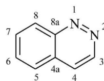
(8) cynolina (PIN)
