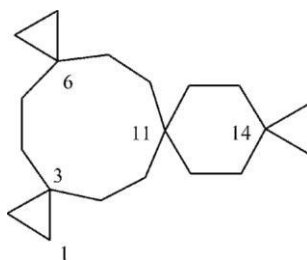
tetraspiro[2.2.2 6 .2.2.2 14 .2 11 .2 3 ]ikozan niepoprawnie
