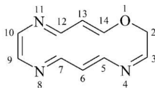
2H-1,4,8,11-oksatriazacyklotetradecyn
