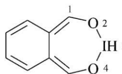
3H - 3\lambda^3,2,4 -benzoidadioksepin (PIN)
