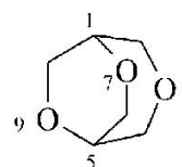
3,7,9-trioksabicyklo[3.2.2]nonan
