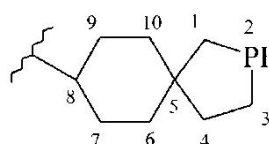
2-fosfasp[4.5]dekan-8-yl (preferowany przedrostek)
