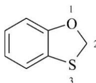
2H-1,3-benzoksatiol (PIN)
