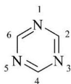
1,3,5-triazyna (PIN)
