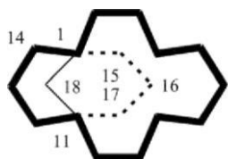
tricyklo[9.3.3.1 1,11 ]oktadekan (PIN)
