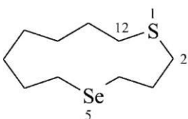
1-tia-5-selenacyklododekan (PIN)
