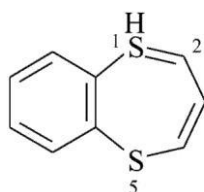
7\lambda^4 -[1,2]ditiolo[5,1- e ]dithiol (PIN)
