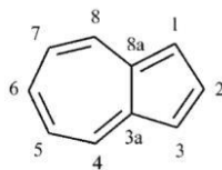
(17) azulen (PIN)
