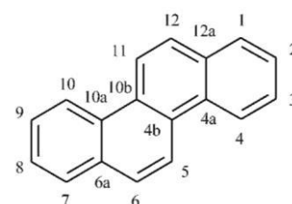
(8) chryzen (PIN)
