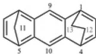
1,4-etano-5,8-metanoantracen (PIN)
