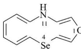
1-oksa-4-selena-11-azacyklotrideka-2,5,7,9,12- pentaen (PIN) 11 H -1-oksa-4-selena-11-aza-[13]annulen
