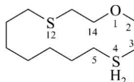
1-oksa-4λ 4 ,12-ditiacyklotetradekan (PIN)
