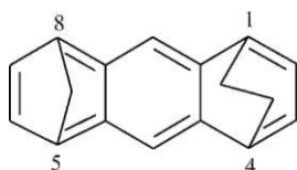
1,4-etano-5,8-metanoantracen (PIN)
