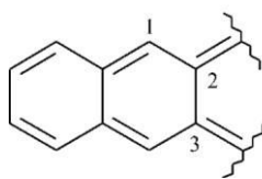
naftaleno-2,3-diylden (preferowany przedrostek)
