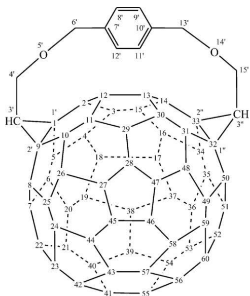
3'H,3''H-3',3''-(metanooksymetano[1,4] benzenometanooksymetano)dicyklopropa[1,9:32,33] ( C_{60}-I_h )[5,6]fulleren (PIN) 1,9:32,33-(etano-1,2,2-triylloksymetyleno-1,4-fenyleno- metylenooksyetano-1,2,2-triyllo)( C_{60}-I_h )[5,6]fulleren
