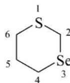
1,3-tiaselenan (PIN)
