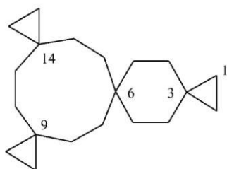
tetraspiro[2.2.2.2 9 .2.2 14 .2.6.2 3 ]ikozan (PIN) poprawnie
