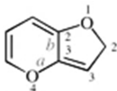
2 H -furo[3,2- b ]piran (PIN) [piran (pierścień 6) preferowany względem furanu (pierścień 5)]
