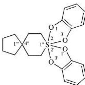
2λ 6 ,2',2''-spiroter[[1,3,2]benzodioxatiol] (PIN)
