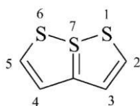
7\lambda^4 -[1,2]ditiolo[5,1- e ]dithiol (PIN)
