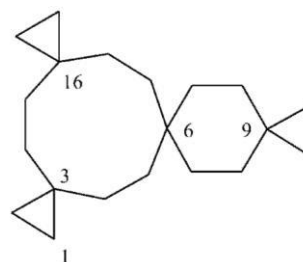
tetraspiro[2.2.2.2 9 .2.2 16 .2.2.2 3 ]ikozan niepoprawnie
