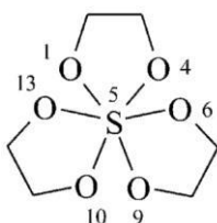
1,4,6,9,10,13-heksaoksa-5λ 6 -tiaspiro[4.4 5 .4 5 ]tridekan (PIN)
