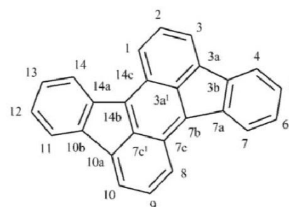
(4) rubicen (PIN)
