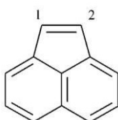
acenaftylen (PIN)
