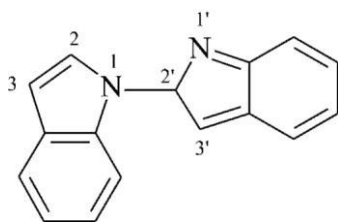
2' H -1,2'-biindol (PIN)
