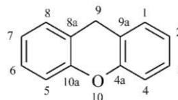
(22) ksanten (specjalna numeracja; pokazano izomer 9 H ; PINem jest 9 H -ksanten) tioksanten (S zamiast O) (specjalna numeracja; pokazano izomer 9 H ; PINem jest: 9 H -tioksanten) selenoksanten (Se zamiast O) (specjalna numeracja; pokazano izomer 9 H ; PINem jest: 9 H -selenoksanten) telluroksanten (Te zamiast O) (specjalna numeracja; pokazano izomer 9 H ; PINem jest: 9 H -telluroksanten)
