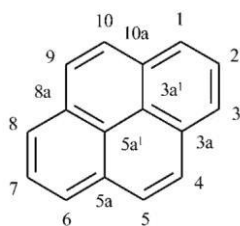
(9) piren (PIN)
