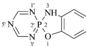
3H-2λ 5 -spiro[[1,3,2]benzoksazafosfol-2,2'-[1,3,5,2]triazafosfinin] (PIN)
