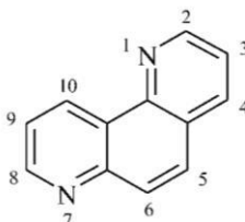
(2) fenantrolina
