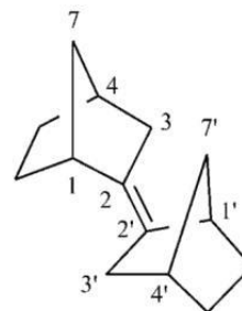
2,2'-bi(bicyklo[2.2.1]heptanylidene) (PIN) (nie \Delta^{2,2'} -bicyklo[2.2.1]heptanylidene)
