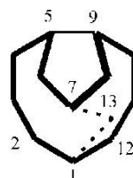
tricyklo[5.5.1.0 5,9 ]tridekan niepoprawnie
