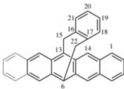
6,13-(metano[1,2]benzenometano)pentacen (PIN)
