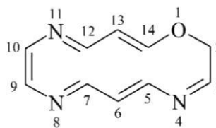
2H-1,4,8,11-oksatriazacyklotetradekyn 1-oksa-4,8,11-triazacyklotetradeka-3,5,7,9,11,13-heksaen (PIN)
