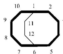
bicyklo[4.4.2]dodekan (PIS)
