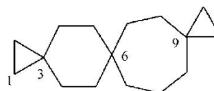
trispiro[2.2.2.2 9.3 6.2 3 ]heksadekan niepoprawna
