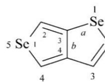
selenofeno[3,4- b ]selenofen (PIN)
