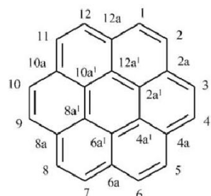
(3) koronen (PIN)
