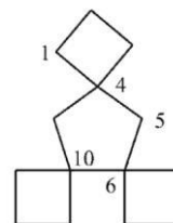
trispiro[3.1.3 6 .0.3 10 .1 4 ]tetradekan niepoprawnie
