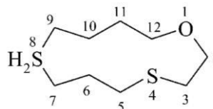
1-oksa-4,8 \lambda^4 -ditiacyklododekan (PIN)
