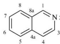
(14) izochinolina*† (PIN)
