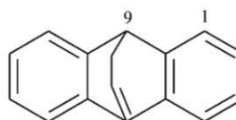
9H-9,10-(epietanyloylideno)antracen (PIN) [nie 9H-10,9-(epietanyloylideno)antracen; przyrostek '-yl' ma pierwszeństwo w wyborze lokantu przyłączenia do układu pierścieni (patrz P-25.4.3.2.2)]
