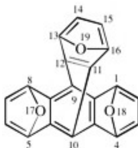
13,16-epoksy-1,4:5,8-diepoksy-9,10-[1,2]benzenoantracen (PIN)
