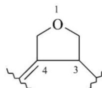
oksolan-3-yl-4-yliden (preferowany przedrostek)
