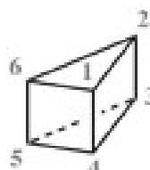
tetracyklo[2.2.0.0 2,6 .0 3,5 ]heksan (nie przyznan)
