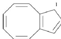
1 H -cyklopenta[8]annulen (PIN)
