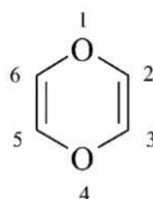
1,4-dioksyn (PIN)
