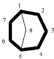
bicyklo[3.2.1]oktan (PIN)
