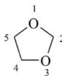
1,3-dioksolan (PIN)
