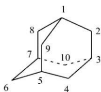
adamantan (PIN) tricyklo[3.3.1.1 3,7 ]dekan
