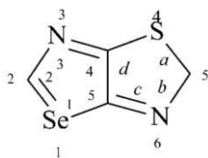
[1,3]selenazolo[5,4- d ][1,3]tiazol (PIN) (S, N starsze od Se, N)
