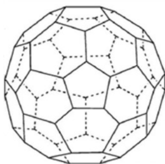
( C_{60}-I_h )[5,6]fulleren (PIN)
