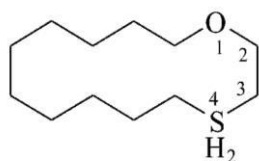
1-oksa-4 \lambda^4 -tiacyklotetradekan (PIN)
