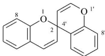
2,4'-spirobi[[1]benzopiran] (PIN) 2,4'-spirobi[chromen]
