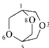
3,6,8-trioksabicyklo[3.2.2]nonan (PIN)
