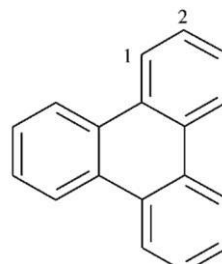
trifenylen (PIN)
