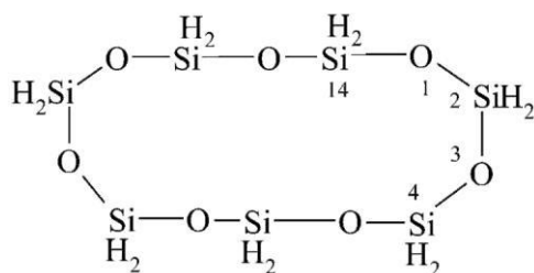
cykloheptasiloksan
