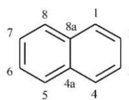
(18) naftalen (PIN)
