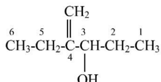
(1) 4- metylidenoheksan-3-ol (PIN)
