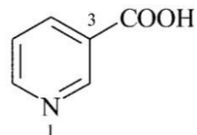
kwasy pirydyno-3-karboksylowy (PIN)
