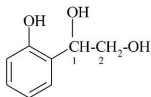
1-(2-hydroksyfenylo)etano-1,2-diol (PIN) [nie 2-(1,2-dihydroksyetylo)fenol; dwie grupy główne są starsze niż jedna]
