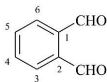
ftaloaldehyd
