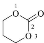
1,3-dioksan-2-on (PIN)
