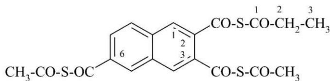
tris(tioanhydryd) 3,6-dioctowo-2-propanowo-naftaleno-2,3,6-trikarboksylowy (PIN)
