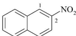
2-nitronaftalen (PIN)
