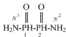
diamid hypodifosfonowy
