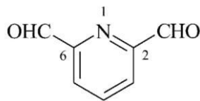
pirydyno-2,6-dikarboaldehyd (PIN)
