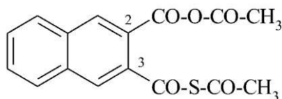
anhydryd 3-[(acetylosulfanylo)karbonyl]naftaleno-2-karboksylowo-octowy (PIN)
