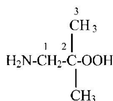
1-amino-2-metylopropano-2-peroksol (PIN)
