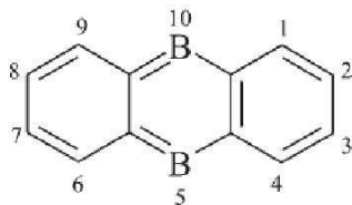
borantren (PIN)
