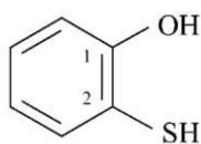
2-sulfanylofenol (PIN)
