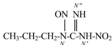
N' -nitro- N -nitroso- N -propyloguanidyna (PIN)
