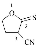
2-sulfanylidenooksolano-3-karbonitryl (PIN)
