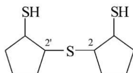
2,2'-sulfanodiylo-di(cyklopentano-1-tiol) (PIN)
