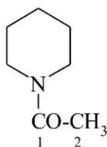
(b) 1-(piperdyn-1-ylo)etan-1-on (PIN) 1-acetylopiperydyna (‘ukryty amid’)
