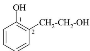
2-(2-hydroksyetylo)fenol (PIN) 2-(2-hydroksyfenylo)etan-1-ol (pierścień jest starszy względem łańcucha w preferowanej nazwie, patrz P-52.2.9)
