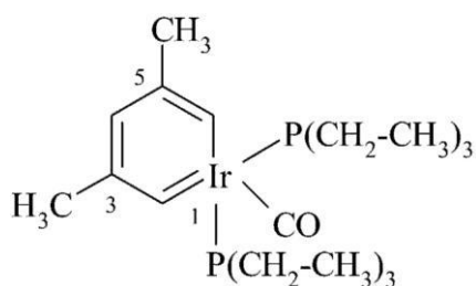
1-karbonylo-3,5-dimetylo-1,1-bis(trietylofosfano)-1-irydabenzen (nazwa zamienna szkieletu)
