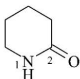
(a) piperdyn-2-on (PIN)
