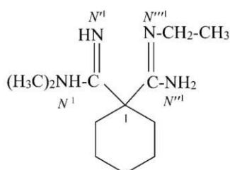
N'''^1 -etylo- N^1, N^1 -dimetylocykloheksano-1,1-dikarboksyimidoamid (PIN)
