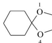
1,4-dioksaspiro[4.5]dekan (PIN) ketal etylenowy cykloheksanonu
