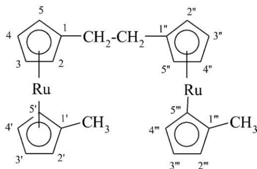
1,1''-(etano-1,2-diyl)bis(1'-metylorutenocen) (PIN)
