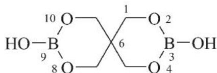
2,4.8.10-tetraoksa-3,9-diboraspiro[5.5]undekano-3,9-diol (PIN)
