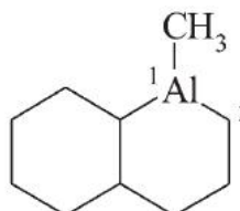
1-metyłodekahydro-1-benzoaluminin
