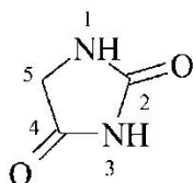
imidazolidyno-2,4-dion (PIN) (nie 2-pirolidon)
