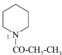
1-(piperydyn-1 ylo)propan-1-on (PIN) 1-propanoilopiperydyna 1-(1-oksopropylo)piperydyna (ukryty amid)
