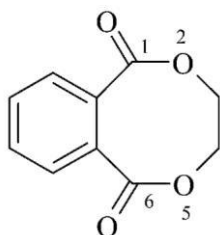
1,3-dioksan-2-on (PIN)
