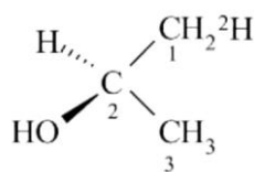
(2R)-(1- 2 H 1 )propan-2-ol (PIN)
