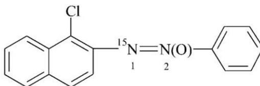
2-oksyl 1-(1-chloronaftalen-2-ylo)-2-fenylo(1- ^{15}\text{N} )diazenu 1-chloro-2-(fenylo-ON ^{15}\text{N} -azoksy)naftalen
