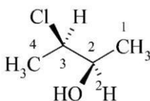
(2R,3R)-3-chloro(2- 2 H 1 )butan-2-ol (PIN)
