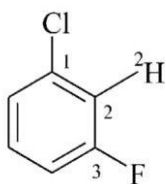
1-chloro-3-fluoro(2- 2 H 1 )benzen (PIN)
