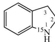
2,3-dihydro( 15 N)-1 H -indol (PIN)
