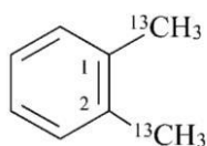
1,2-di[( 13 C)metylo]benzen (PIN) ( \alpha,\alpha' - 13 C 2 )-1,2-ksylen ( \alpha,\alpha' - 13 C 2 )- o -ksylen
