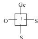
uproszczony digraf dla sfery I
