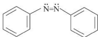
(Z)-difenylodiazen (PIN) (nie cis -difenylodiazen)
