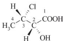
kwas (2 S ,3 S )-3-chloro-2-hydroksybutanowy (PIN)
