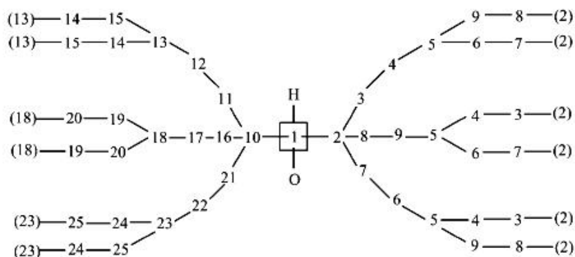
uproszczony digraf
