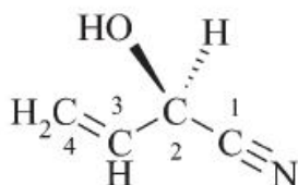
(2 R )-2-hydroksybut-3-enonitryl (PIN)
