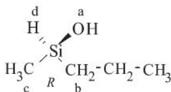
(R)-metylo(propylo)silanol (PIN)
