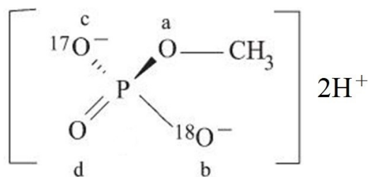
( S )-[ O -metylo( 17 O 1 , 18 O 1 )fosforan] diwodoru (PIN)
