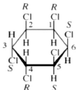
1 (1 R ,2 R ,3 S ,4 R ,5 S ,6 S )
