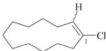
(1 E )-1-chlorocyklododek-1-en (PIN)
