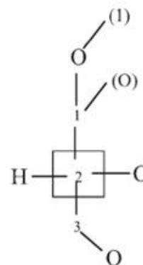
uproszczony digraf
