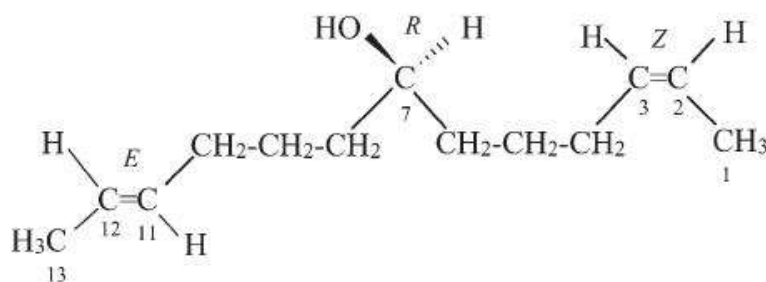
(2 Z ,7 R ,11 E )-trideka-2,11-dien-7-ol (PIN)
