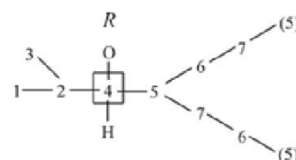
uproszczony digraf
