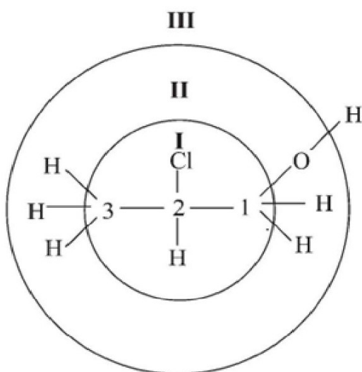
kompletny digraf dla centrum 2
