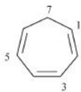
cyklohepta-1,3,5-trien (PIN)
