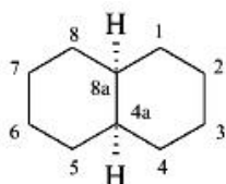
(4a s ,8a s )-dekahydronaftalen (PIN) cis -dekahydronaftalen
