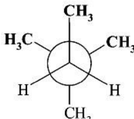
synklinalna
