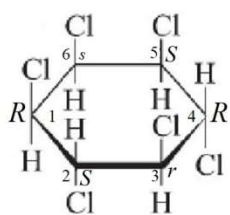
3 (1 R ,2 S ,3 r ,4 R ,5 S ,6 s )
