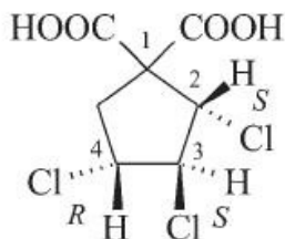
kwas (2 S ,3 S ,4 R )-2,3,4-trichlorocyklopentano-1,1-dikarboksylowy (PIN)
