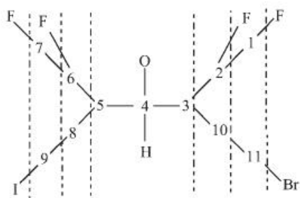
uproszczony digraf
