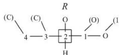
uproszczony digraf
