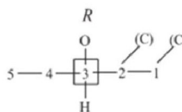
uproszczony digraf
