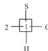
uproszczony digraf dla sfery I
