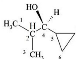
numercacja do digrafu
