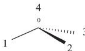
( T-4 ) (pokazano atom fantomalny '0')
