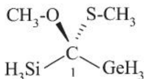
[(R)-germanylo(metoksy)(metylosulfanylo)metylo]silan (PIN) (lokant '1' podany jest jedynie na użytek digrafu ; przy tworzeniu nazwy nie jest on potrzebny)
