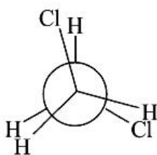
antyklinalna
