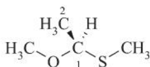
(1R)-1-metoksy-1-(metylosulfanylo)etan (PIN)
