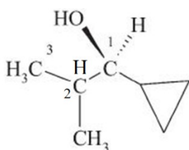
(1R)-1-cyklopentylo-2-metylopropan-1-ol (PIN)
