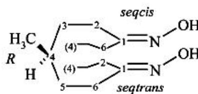
C-4
