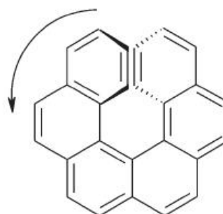
(M)-heksahelicen (PIN)
