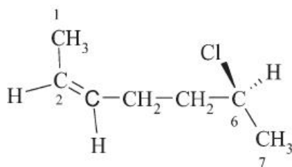
(2 Z ,6 S )-6-chlorohept-2-en (PIN) (numerowanie – patrz P-14.4)
