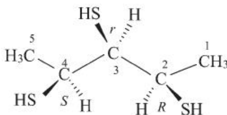
(2 R ,3 r ,4 S )-pentano-2,3,4-tritoliol (PIN)
