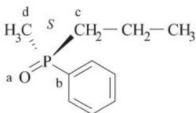
( S )-fenylo(metylo)propylo-λ 5 -fosfanon (PIN; patrz P-74.2.1.4) oksyd ( S )-fenylo(metylo)propylofosfanu
