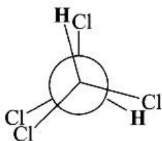
antyklinalna
