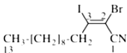
(2 Z )-2-bromo-3-jodotridec-2-enonitryl (PIN)
