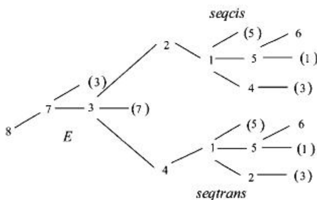
uproszczony digraf
