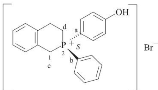
bromek (2 S )-2-fenylo-2-(4-hydroksyfenylo)-1,2,3,4-tetrahydroizofosfinolin-2-ium (PIN)
