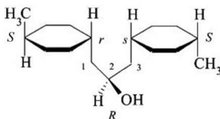
(2R)-1-[(1r,4S)-4-metylocykloheksylo]-3-[(1s,4S)-4-metylocykloheksylo]propan-2-ol (PIN) (2R)-1-( cis -4-metylocykloheksylo)-3-( trans -4-metylocykloheksylo)propan-2-ol
