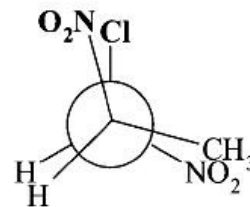
synperiplanarna
