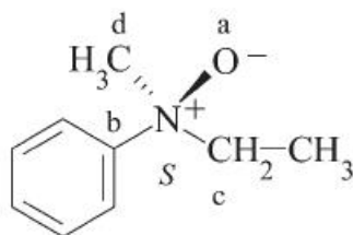
N -oksyd ( S )- N -etylo- N -metyloaniliny (PIN; patrz P-74.2.1.2) ( S )-(N-etylo- N -metyloaniliniumylo)oksydanid
