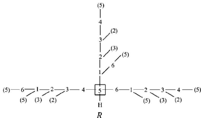
uproszczony digraf
