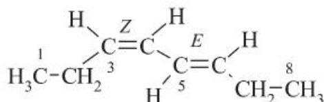
(3Z,5E)-okta-3,5-dien (PIN)
