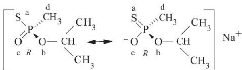
( R )-(metylofosfonotian O -propan-2-ylu)-sodu (PIN)
