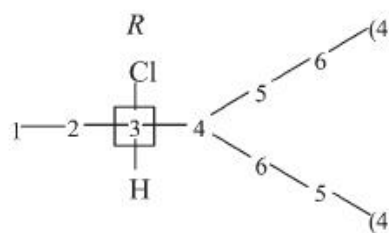
digraf uproszczony
