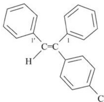
1,1'-[(1 E )-1-(4-chlorofenylo)eteno-1,2-diyl]dibenzen (PIN, patrz P-93.6) 4-chloro-1,1'-[(1 E )-1-fenyloeteno-1,2-diyl]dibenzen
