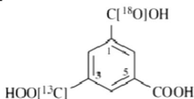
kwas 3-[ 13 C]karboxy-5-karboxybenzeno-1-[ 18 O]karboxylowy (PIN)
