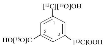
kwas 3-[ 13 C]karboxy-5-[ 18 O]karboxybenzeno-1-[ 13 C, 18 O]karboxylowy (PIN) (nie kwas benzeno-1,3,5-[1,3- 13 C 2 ,1,5- 18 O 2 ]trikarboxylowy)
