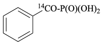
kwask [benzeno( 14 C)karbonylo]fosfonowy (PIN)? kwas [fenylo( 14 C)karbonylo]fosfonowy kwas (karbonylo- 14 C)benzoilofosfonowy
