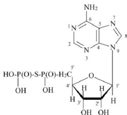
5'-(2-tiodifosforan triwodoru) adenozyliny
