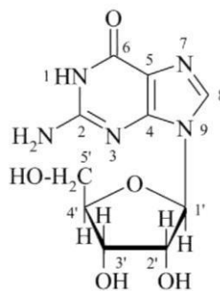
guzanozyna
