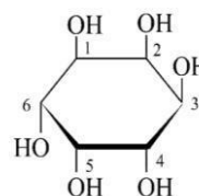
neo -inozyt (1,2,3/4,5,6-)
