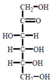
D-fruktoza D- arabino -heks-2-uloza
