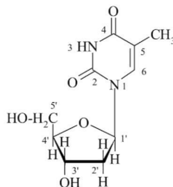
tymidyna
