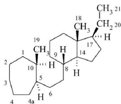
9,10-seko-4a-homo-5 \alpha -pregnan
