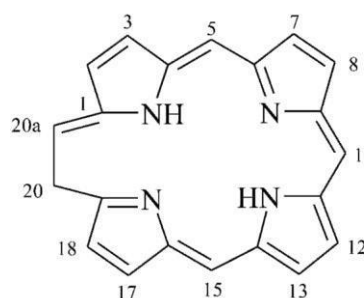
(B) 20H-20a-homoporfiryňa
