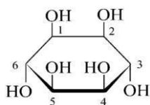
muko -inozytol (1,2,4,5/3,6-)
