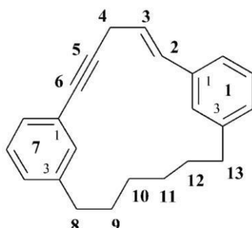
1,7(1,3)-dibenzenacyklotridekafan-2-en-5-yn (PIN)
