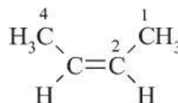
(2Z)-but-2-en (PIN)
